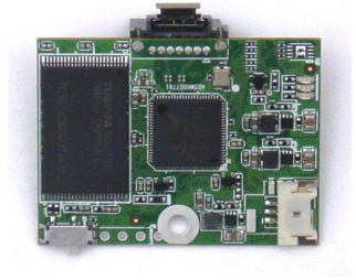
SATA DOM
